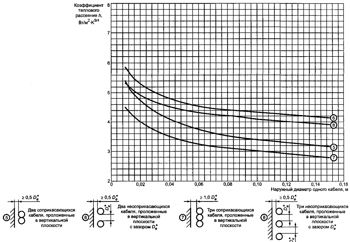
Рисунок 7b - Кoeffициент теплового рассеяния для кабелей с черной поверхностью, проложенных на воздухе
