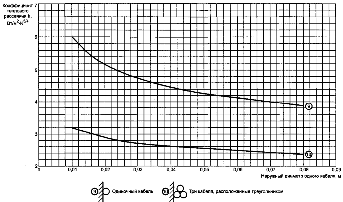
Рисунок 7с - Кoeffициент теплового рассеяния для кабелей с черной поверхностью, проложенных на воздухе
