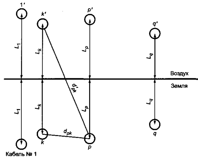
Рисунок 1 - Схема с изображением группы из q кабелей и их отражений в плоскости земля-воздух
