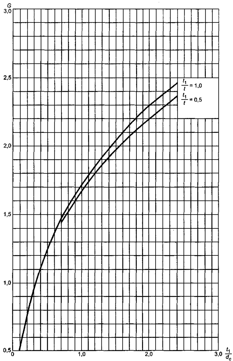
Рисунок 2 - Геометрический фактор G для двужильного кабеля с поясной изоляцией и круглыми жилами (см. 2.1.2.1)
