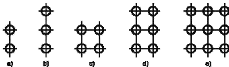
Рисунок 1 — Типовые примеры групп кабелей (e) представляет собой группу самого большого размера, на которую распространяются данные]
