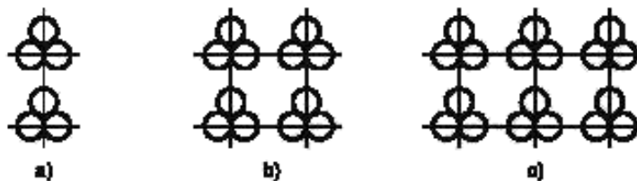
Рисунок 2 — Типовые примеры групп кабелей, проложенных треугольником (c) представляет собой группу самого большого размера, на которую распространяются данные]
