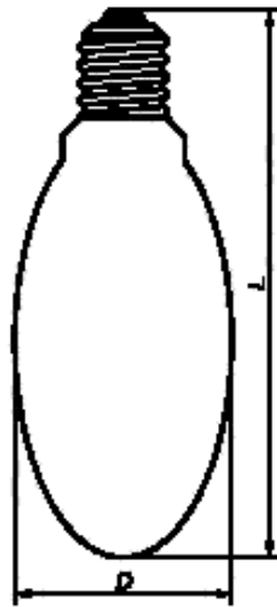
Рисунок 1 — Лампа ртутная высокого давления
