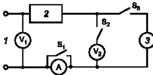
1 — синусоидальный источник питания; 2 — ДОИ; 3 — лампа
