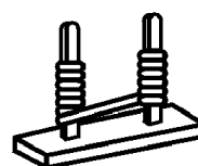
Соединение обжимом
