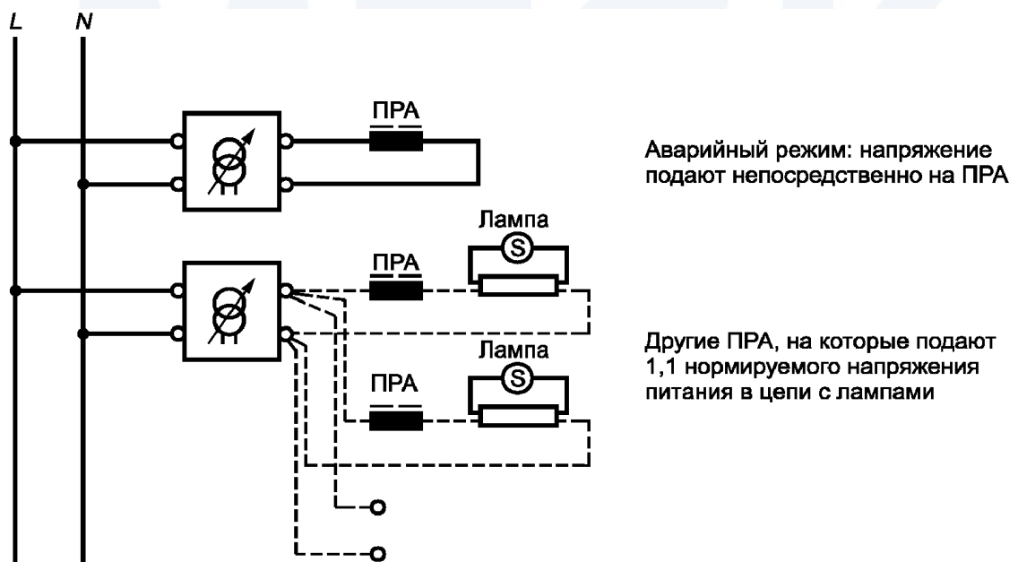
Рисунок 32. Схема испытания светильников с люминесцентными лампами \leq 70 Вт
