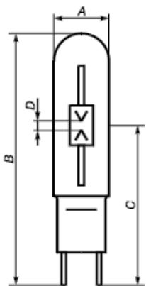
Рисунок 2 - Лампа с цоколем G8.5
