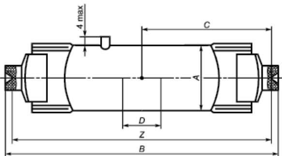
Рисунок 3 - Лампа с цоколями RX7s и RX7s-24
