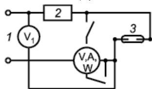
1 - источник питания; 2 - ДООИ; 3 - лампа Рисунок В.1 - Схема
