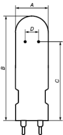
Рисунок 1 - Лампа с цоколем G12
