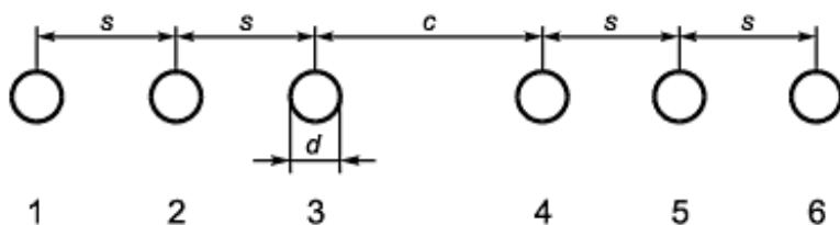
Рисунок 1 - Расположение кабелей
