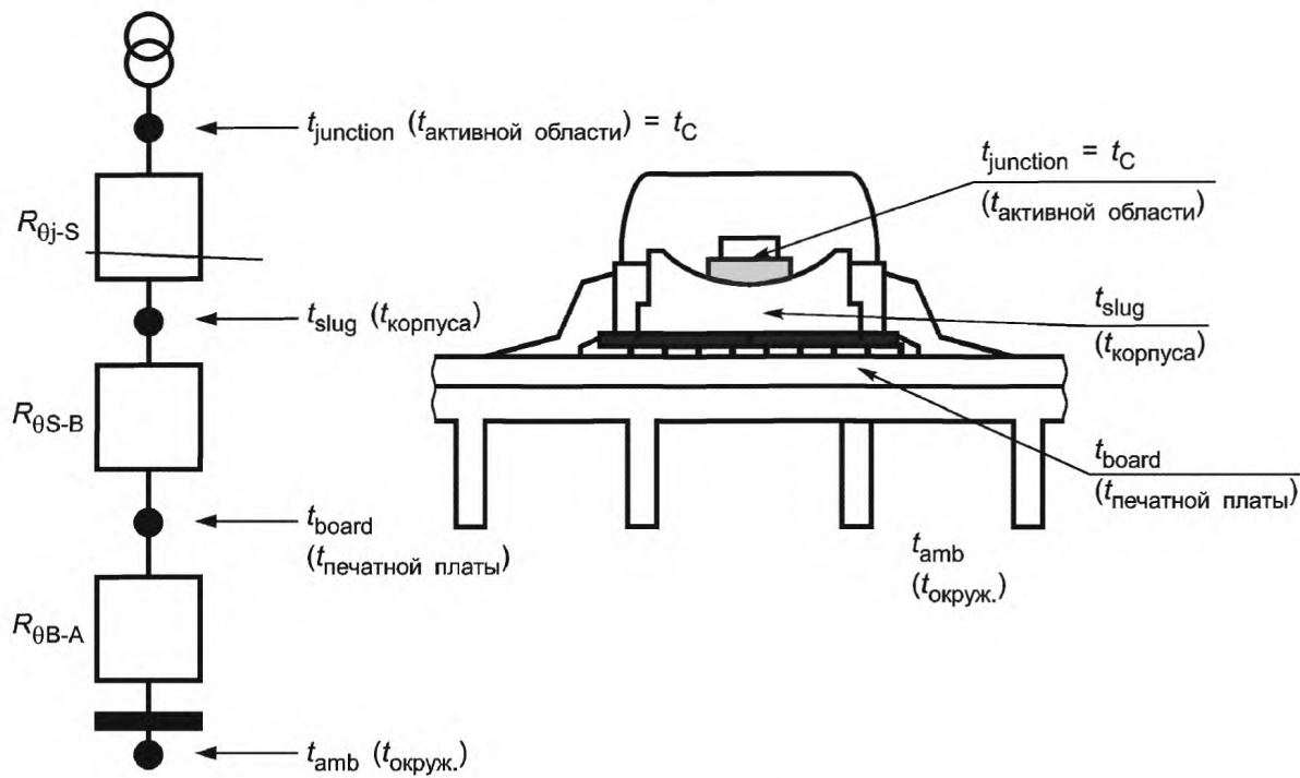
Рисунок 1 — Схематическая цепочка тепловых сопротивлений
